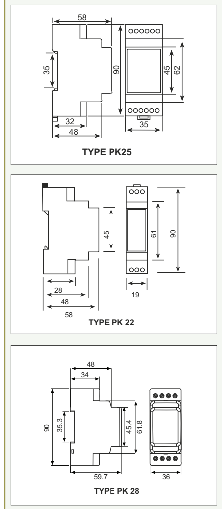
Dimensions
