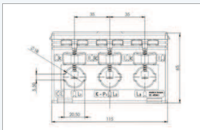
Dimensions
