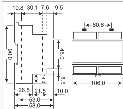
TYPE DIN / PK 26
