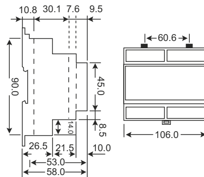
TYPE DIN 4 / PK 26
