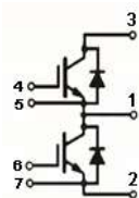
Circuit 1(Phase Leg)
