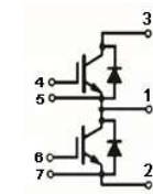
Circuit 1(Phase Leg)
